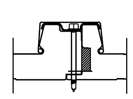
SOLAPE LONGITUDINAL 3
