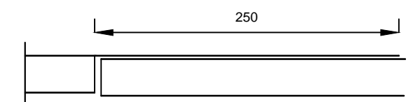
SOLAPE TRANSVERSAL
