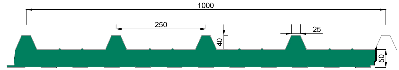
PANEL SÁNDWICH 5 LOMOS LANA DE ROCA
