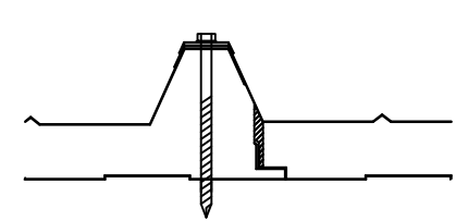
SOLAPE LONGITUDINAL 2
